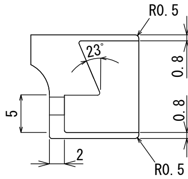
A-A断面図
