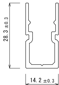
原寸 (1:1)
