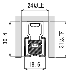
最小施工寸法 (1:2)
