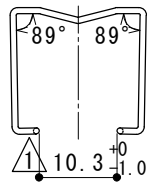
フリー時形状 1/1
